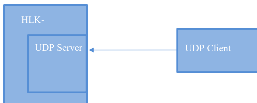
图 14. UDP Server
