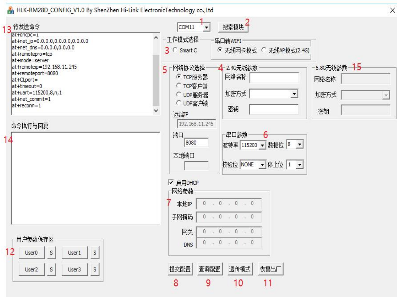
图 24. 串口配置工具界面
