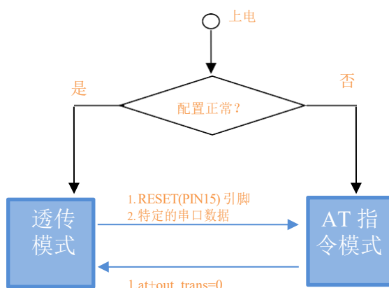
图 10.串口工作状态转换
