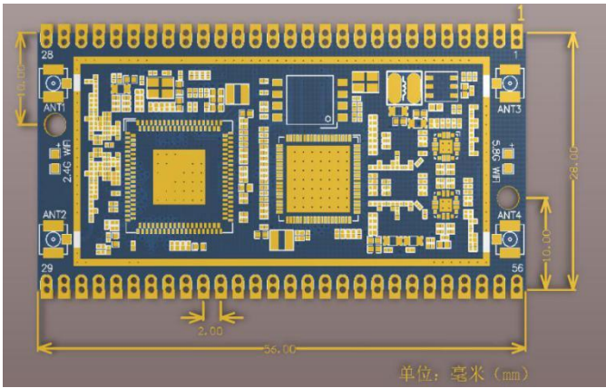
图 1 HLK-RM28E尺寸
