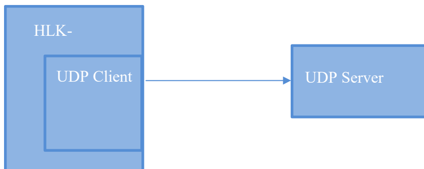
图 15. UDP Client
