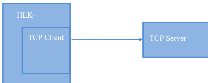
图 13. TCP Client
