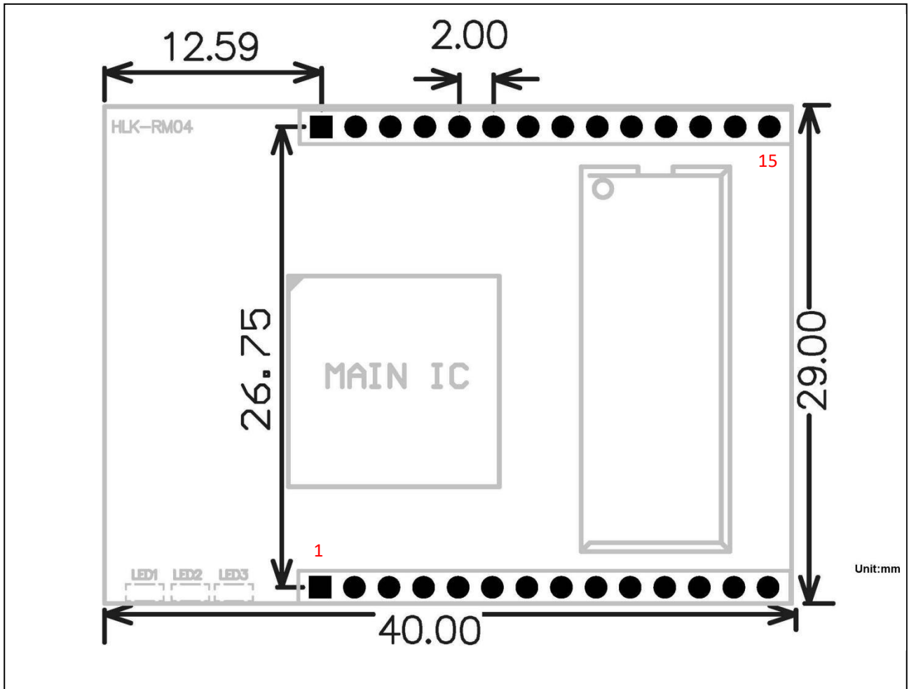
图 2.尺寸 (单位 mm)
