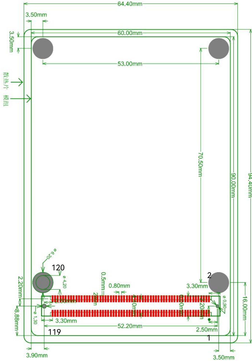
图 9. 封装尺寸
