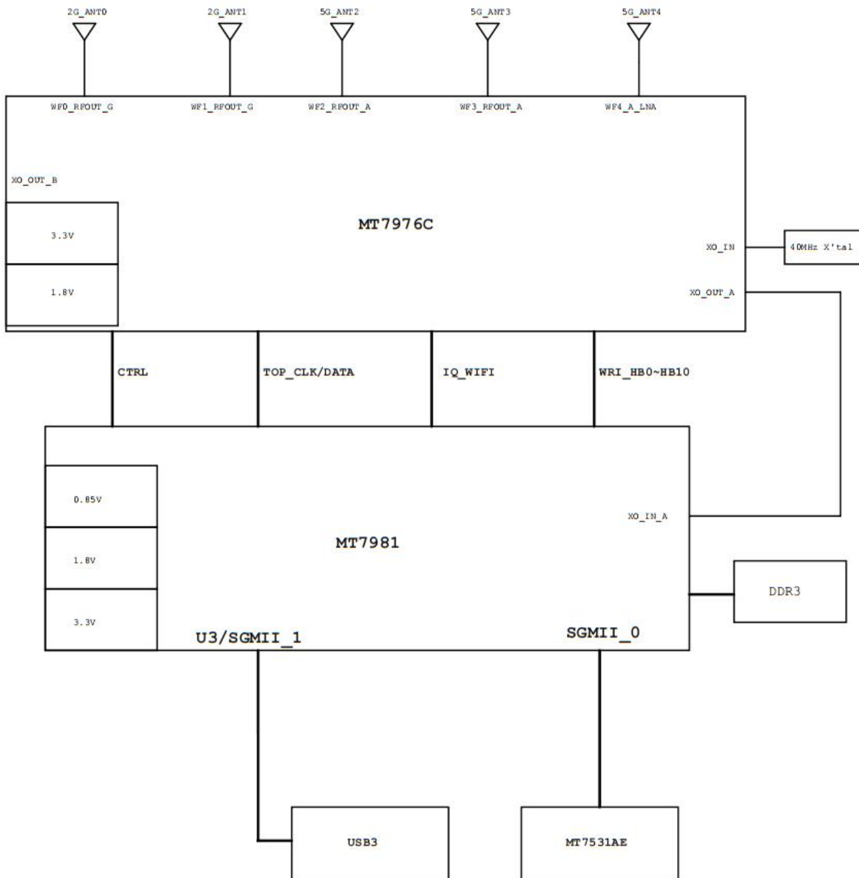
图 1. 方框图
