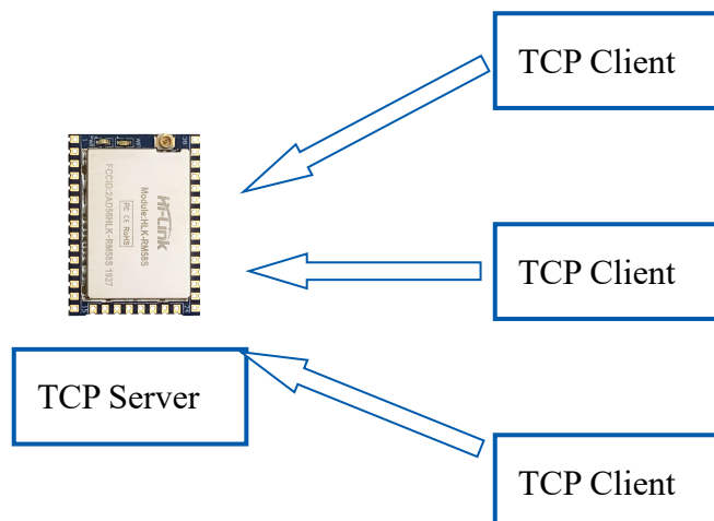
图 10 TCP Server
