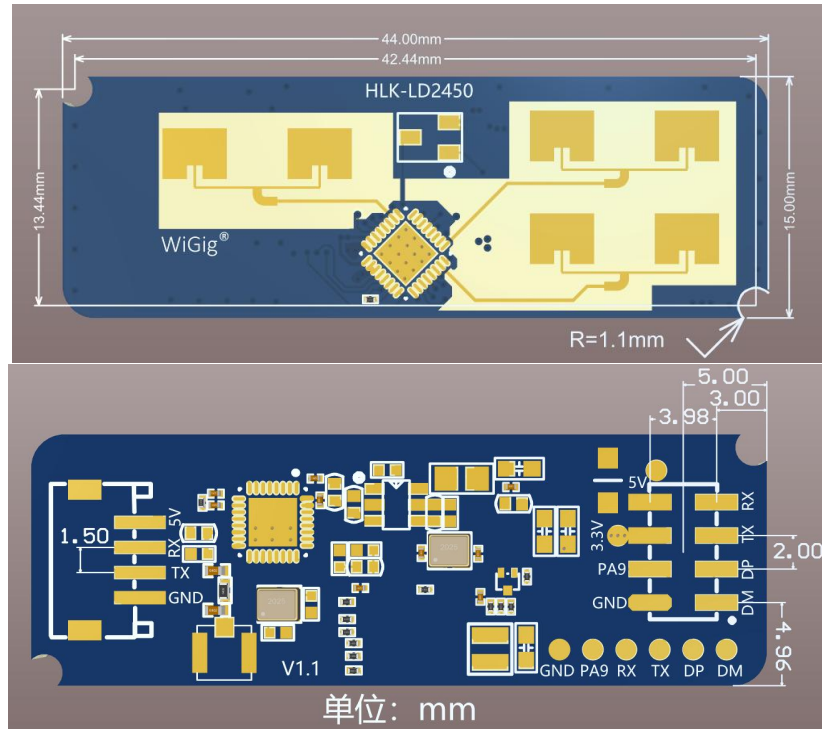
图 3 模块尺寸图
