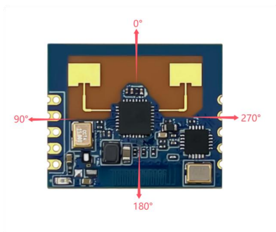
图 7 挂顶安装示意图
