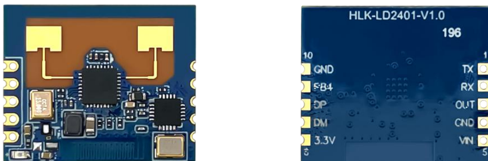
图 4 模块实物图
