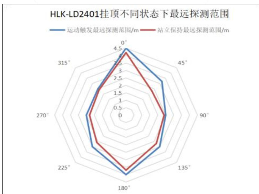
图 8 探测范围示意图(挂顶高度3米)
