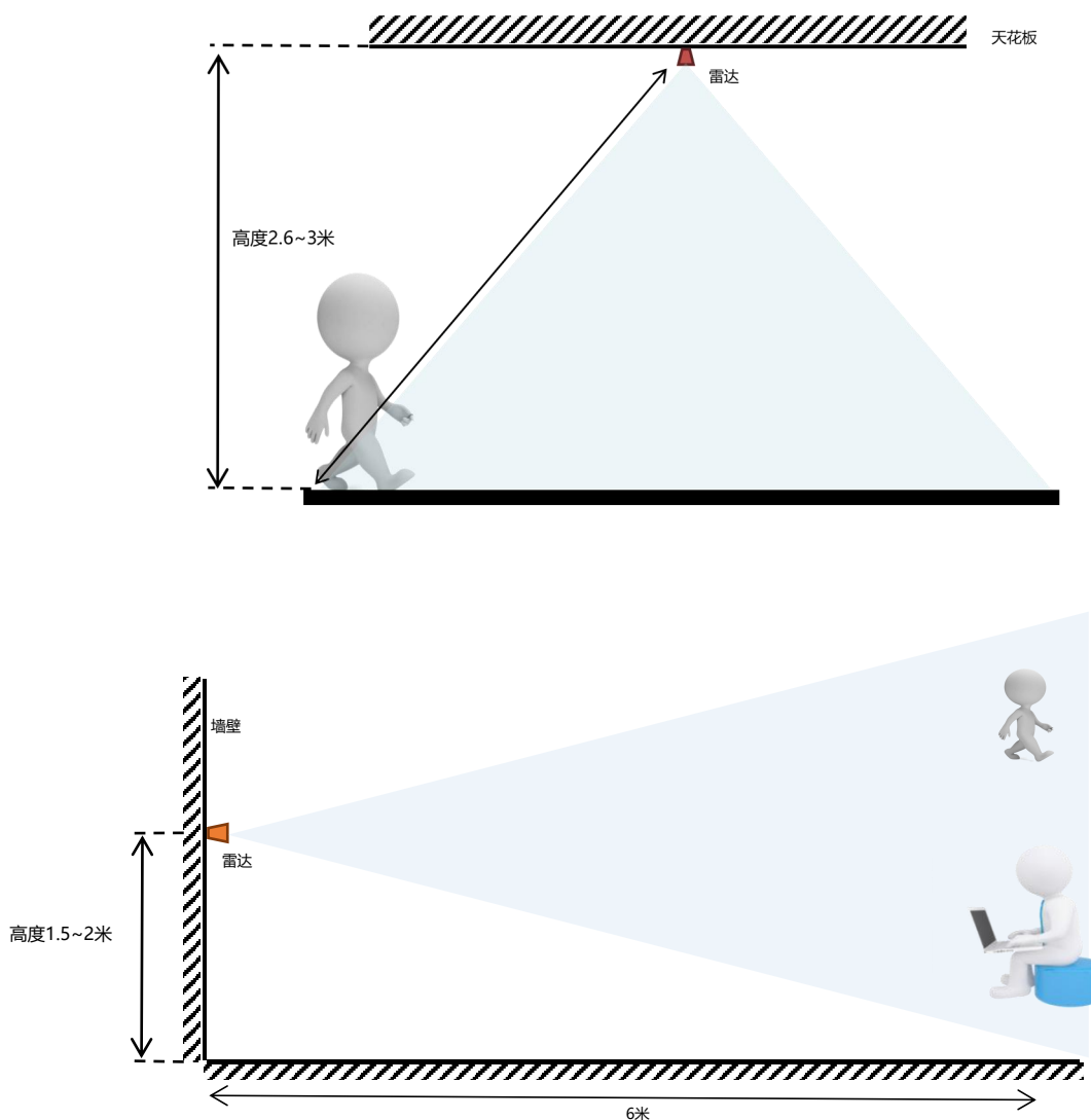
图 1 使用方式图示
