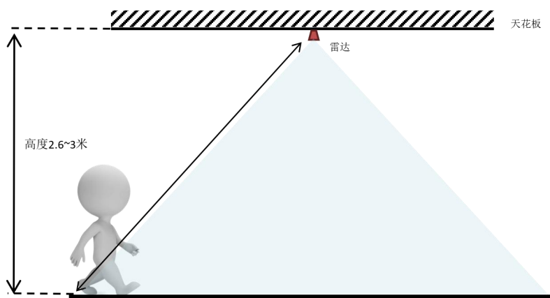
图 7 挂顶安装示意图
