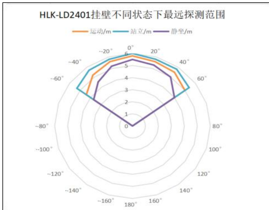
图 10 探测范围示意图(挂壁高度1.5米)
