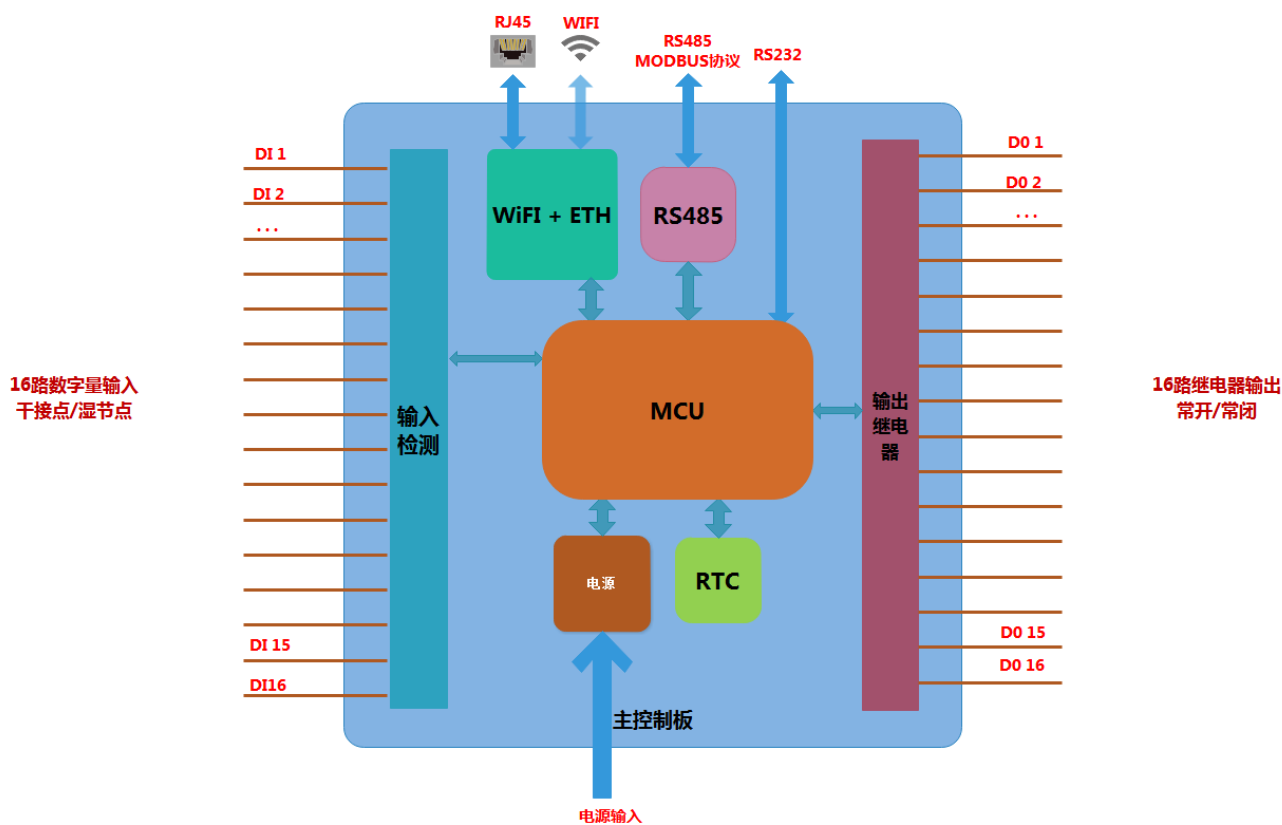
图 1 产品组成框图
