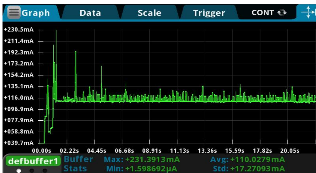
图 24. sta 模式透传电流测试
