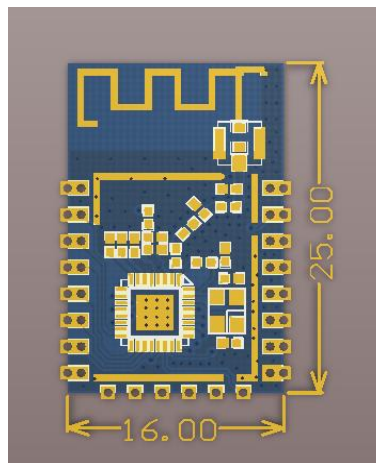
图 1 HLK-B30 封装大小
