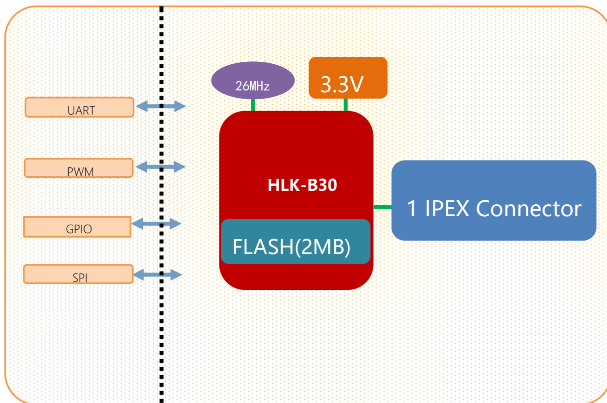
图 2. HLK-B30 模块架构图
