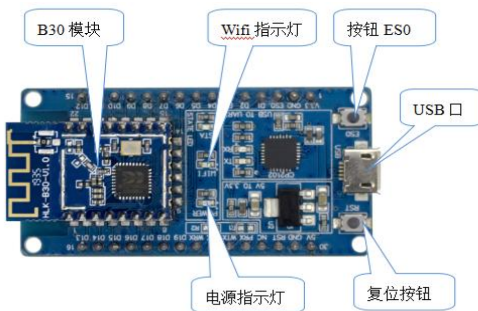
图 3 底板说明图
