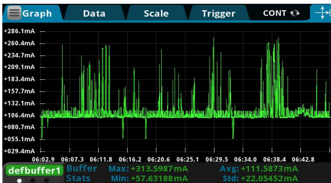
图 22 ap 模式透传电流测试
