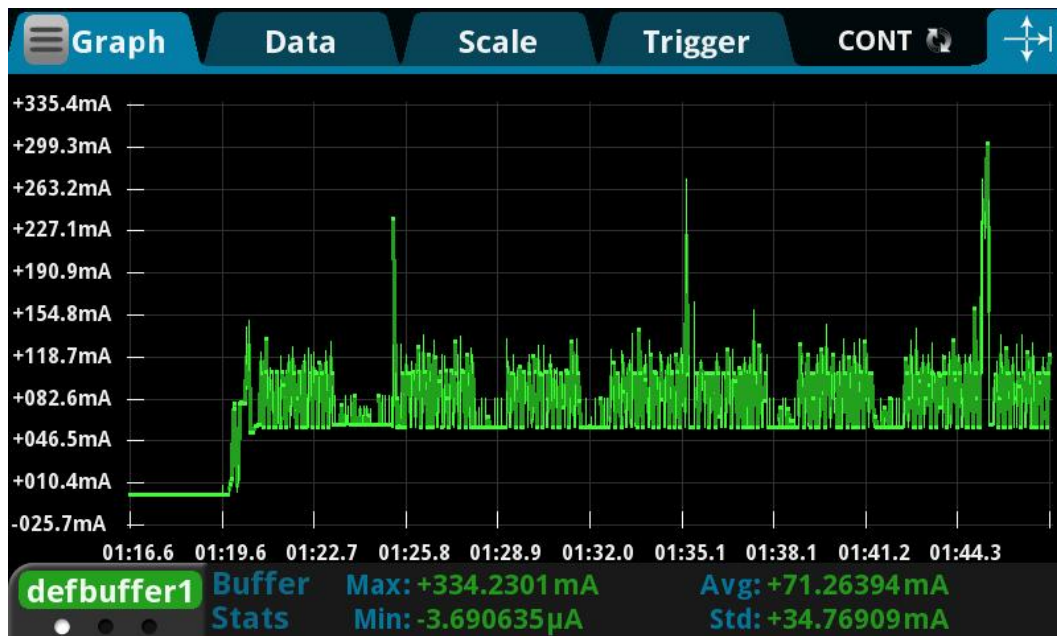
图 25. 默认模式电流测试
