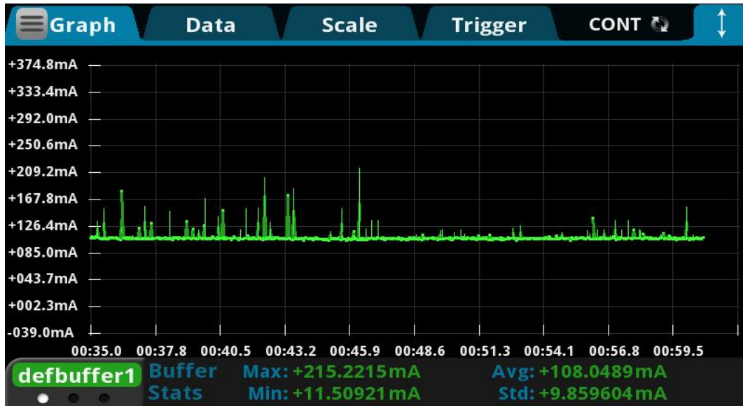
图 23. BLE+WiFi 透传电流测试
