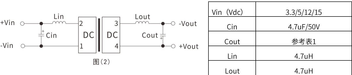
推荐 EMI 参考电路值详（表 2）
