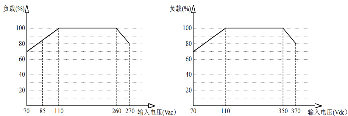
输入电压与负载特性曲线
