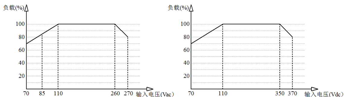
输入电压与负载特性曲线
