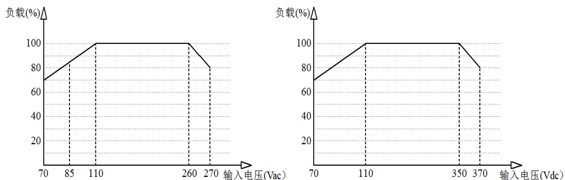
输入电压与负载特性曲线
